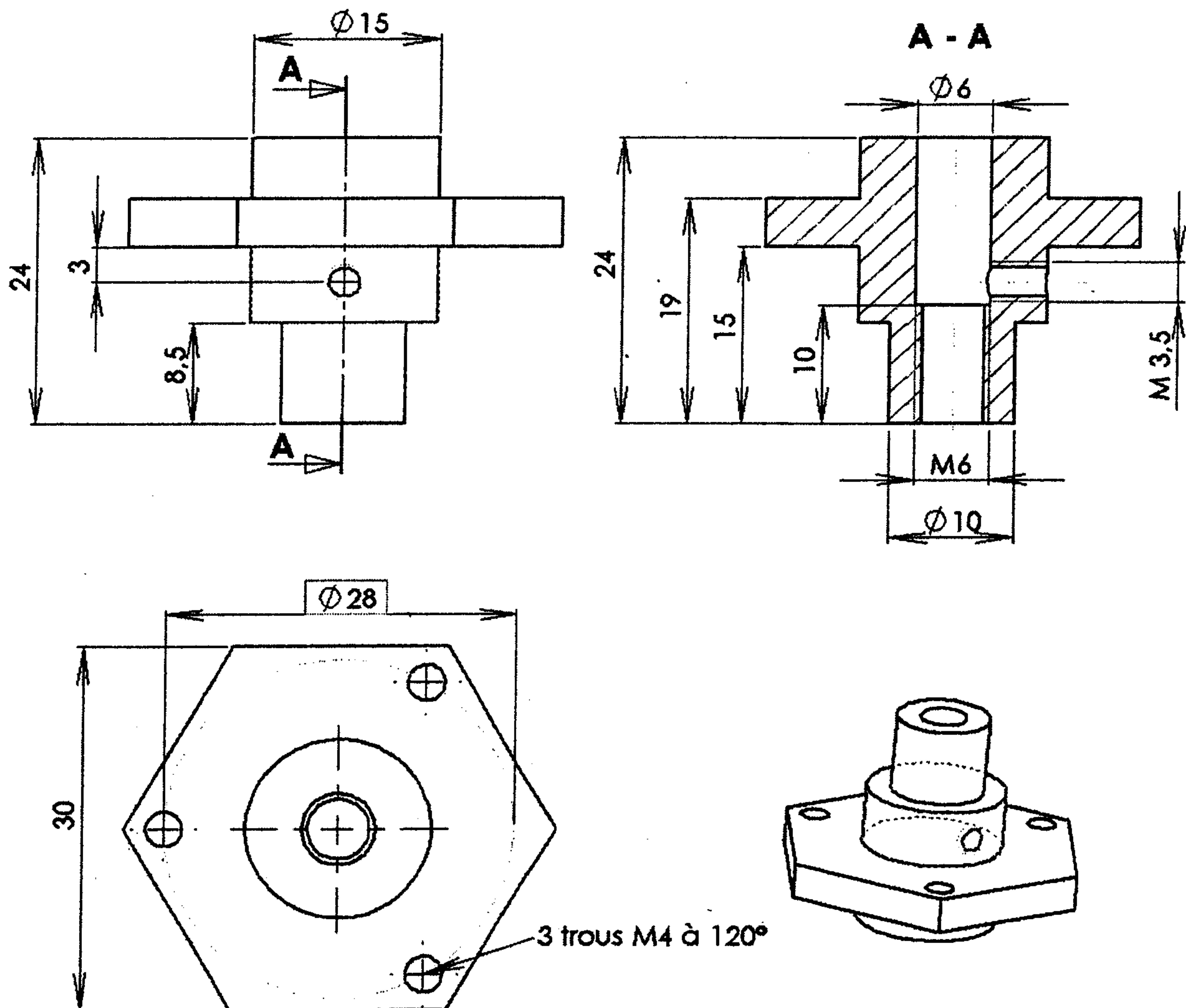
Dessin de définition de l'axe de liaison
