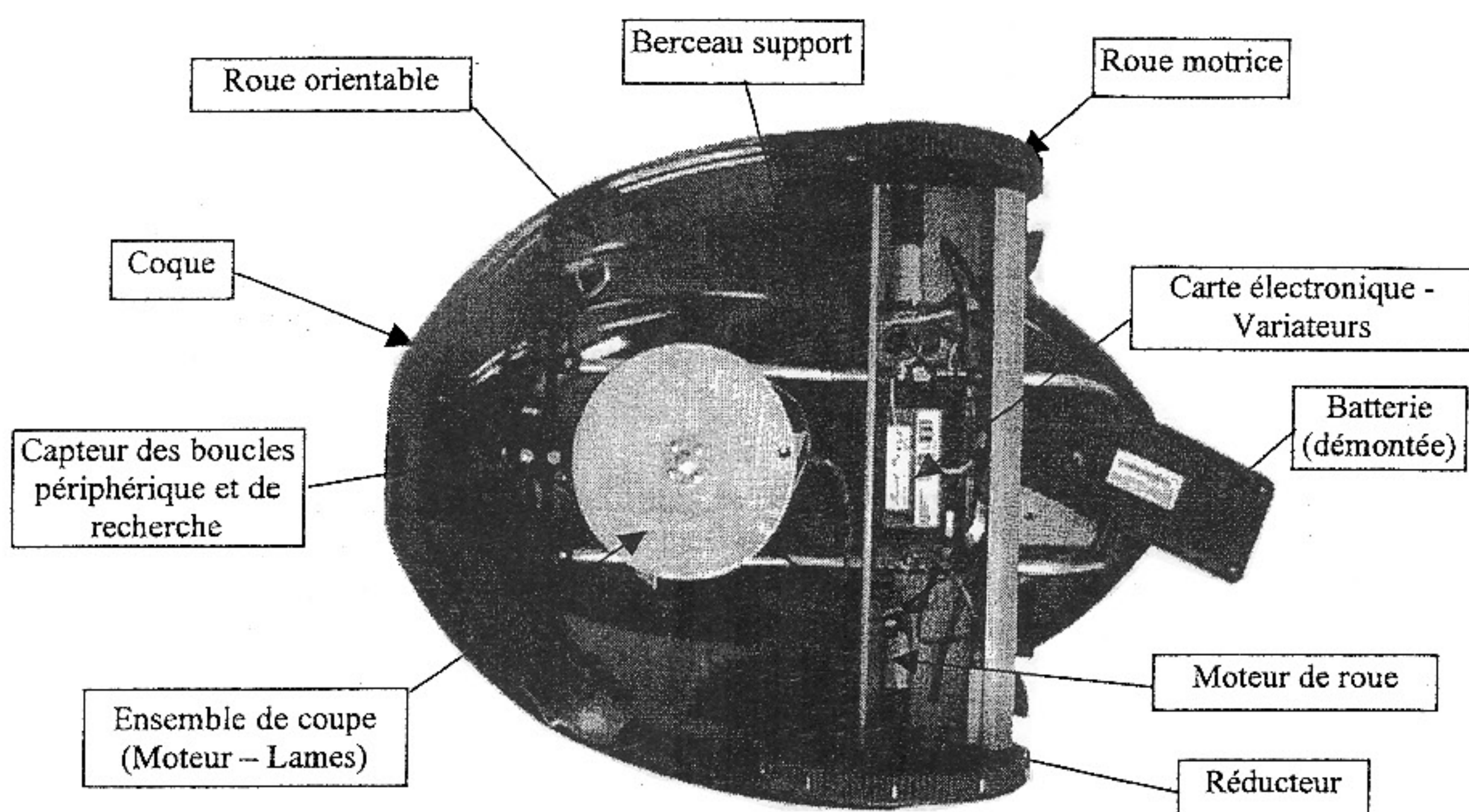
Figure 8 : Vue de dessous
